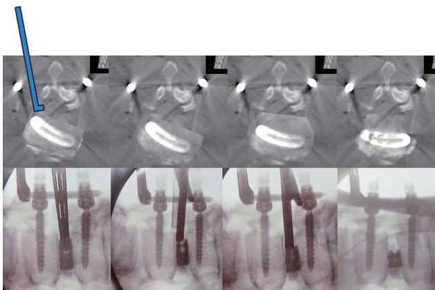
図3 ブーメランケージの挿入方法 (ゲージの水平化)
